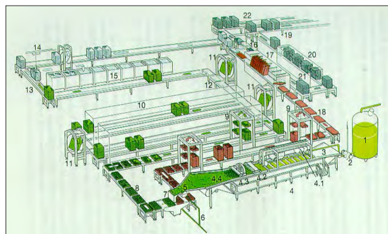
Fabricarea brânzeturilor cu mușcăi la suprafață prin procedeul cu coagulator ALPMA (Fig. 8.18 din capitolul "Brânzeturi cu floră fungică")
