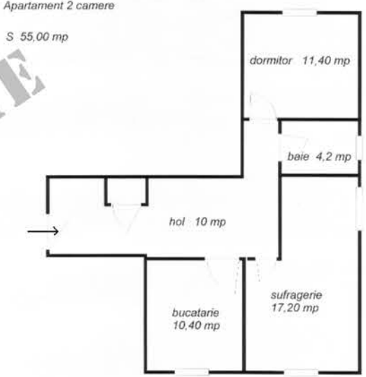
Apartament 2 camere
