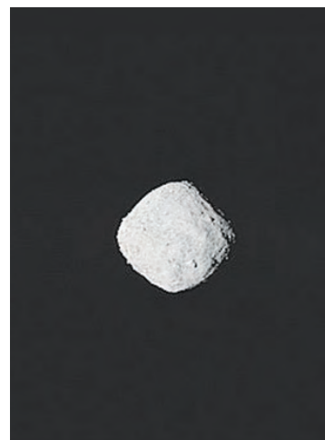
● Bennu
